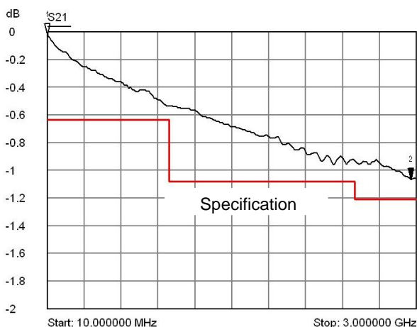
RG223-01-03-1000 的典型 S21 指标:
