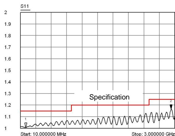
RG223-01-03-1000 的典型 S11 指标:
