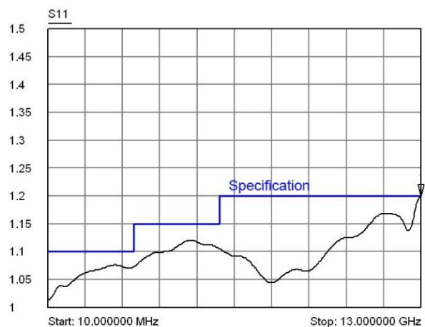
141-01-01-100R 的典型 S11 指标:
