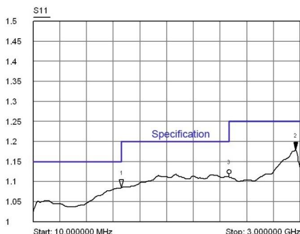
RG214-03-04-1000 的典型 S11 指标:
