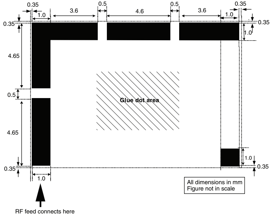
Fig. 6 - VJ 6040 Footprint
