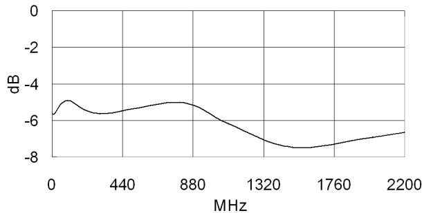
IIP3
