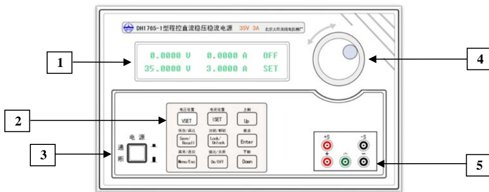
图 5.1 前面板
