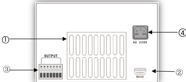
图 5.2-1 后面板
