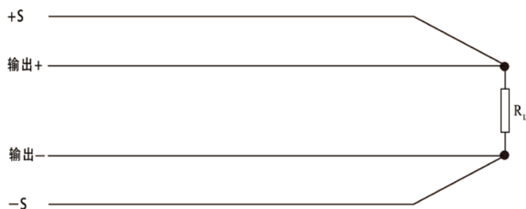
图 5.2-2 远端测量接线方法
