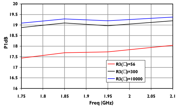
P1dB
