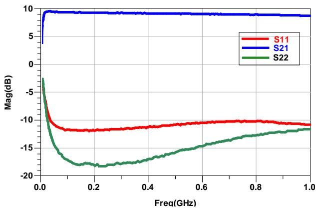
S-Parameter
