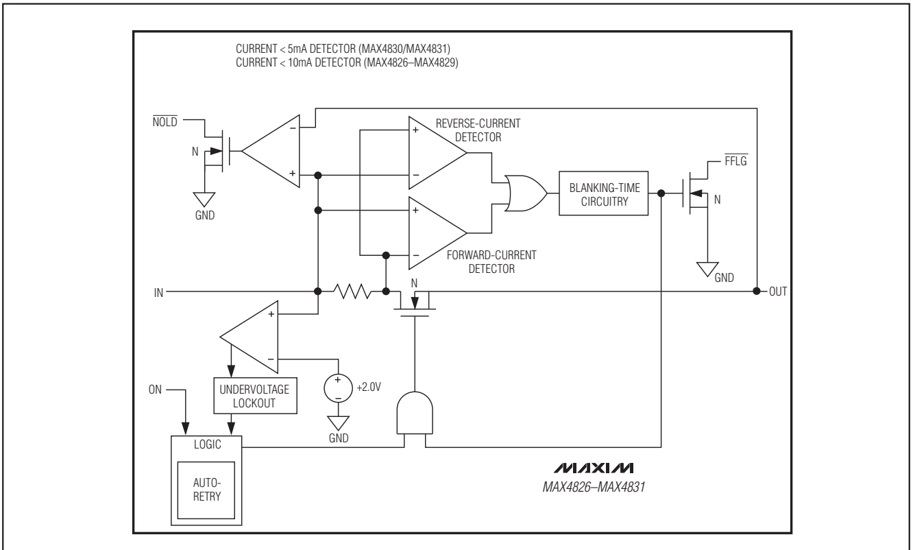
功能框图
