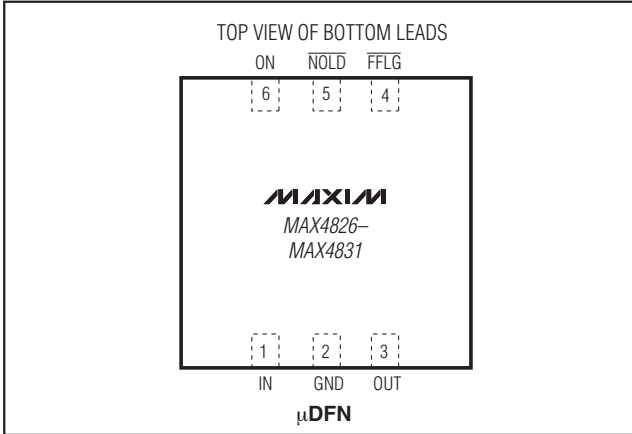
引脚配置
