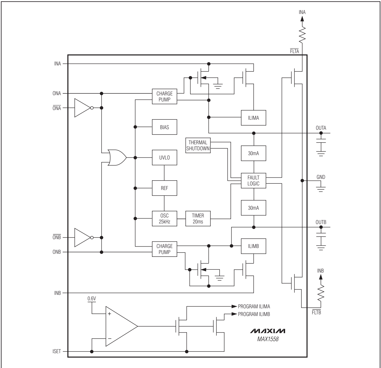
图2. 功能框图
