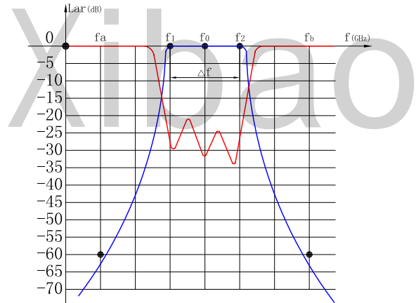
XB-BPF-60dB带通滤波器特性曲线图
