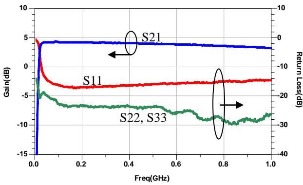
S-Parameter
